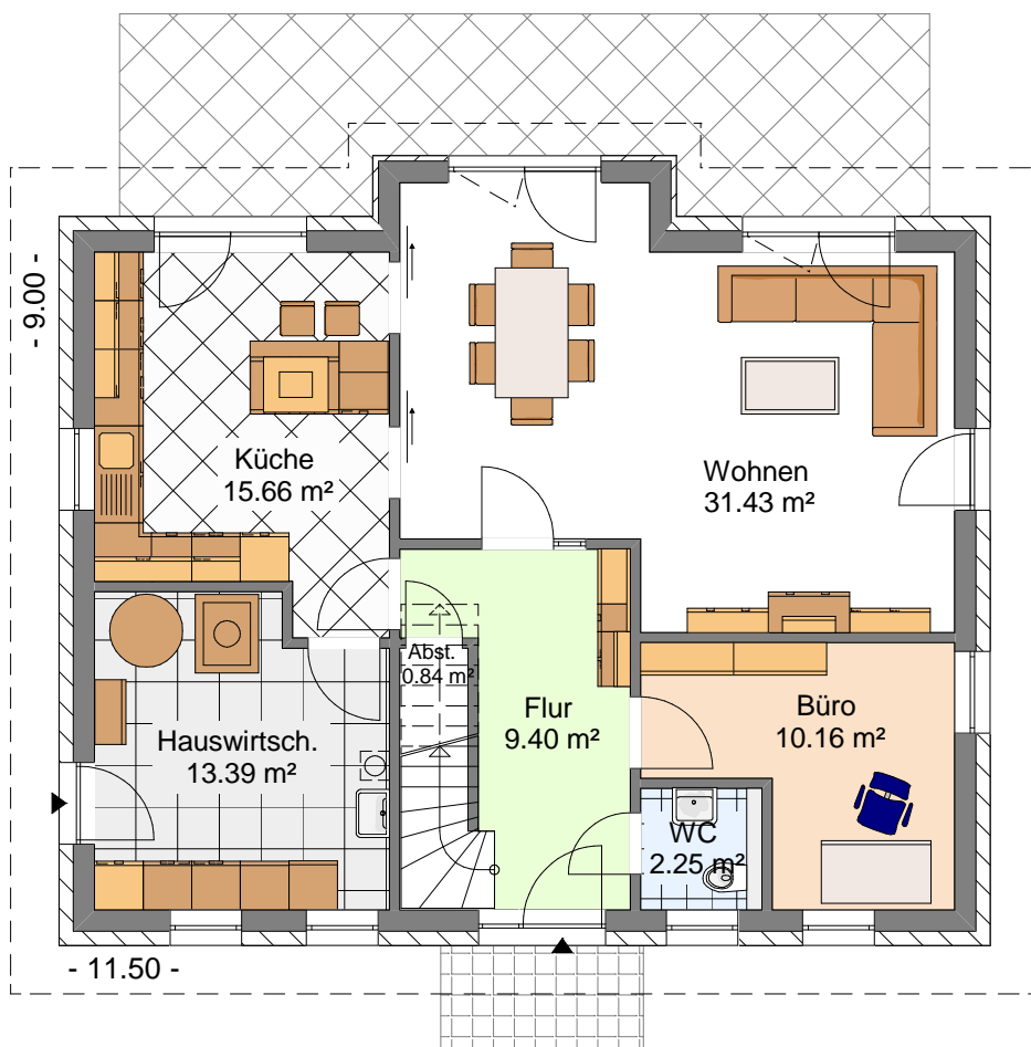
ERDGESCHOSS
