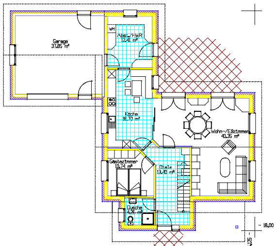
ERDGESCHOSS Wohnfläche: 99,86 m 2 Nutzfläche: 37,85 m 2
