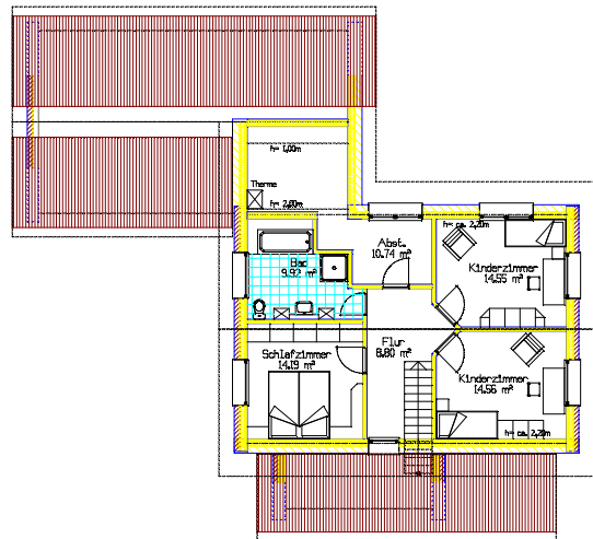
DACHGESCHOSS Wohnfläche: 72,76 m 2
