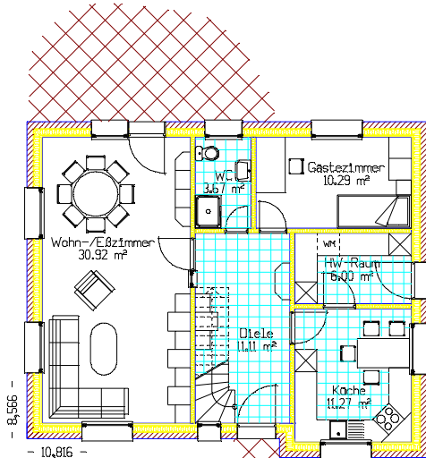
ERDGESCHOSS Wohnfläche: 73,26 m 2
