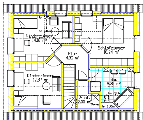
DACHGESCHOSS Wohnfläche: 59,63 m 2
