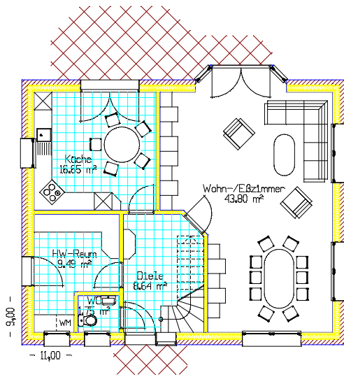
ERDGESCHOSS Wohnfläche: 80,33 m 2
