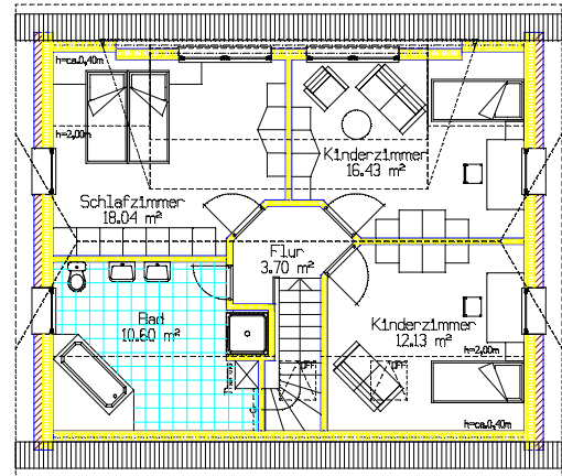
DACHGESCHOSS Wohnfläche: 60,90 m 2
